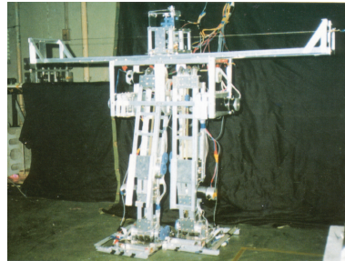
Osaka Univ. Idaten II (1982)
