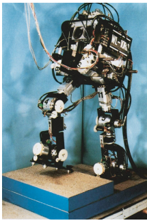
Waseda Univ. WL-10RD (1984)
